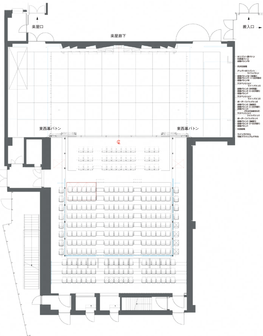
舞台平面図
