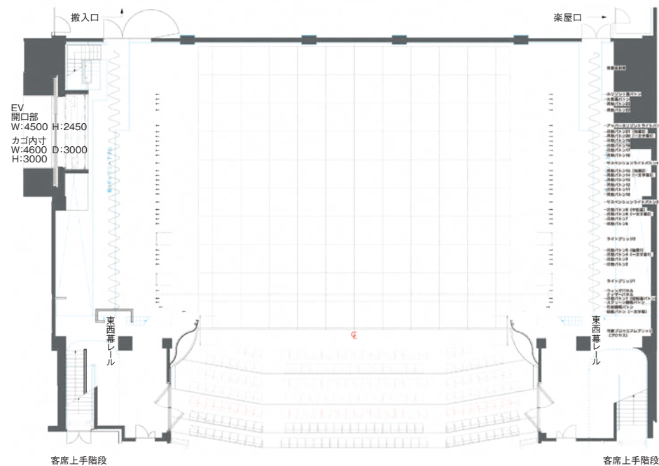
舞台平面図
